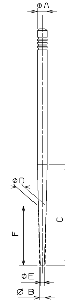
SPILLO BICONICO
